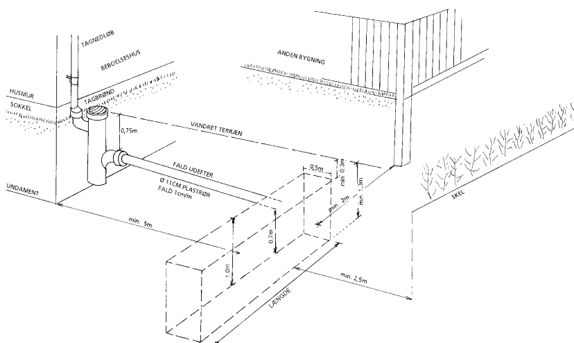
figur 1: Principskitse for placering af faskine.
